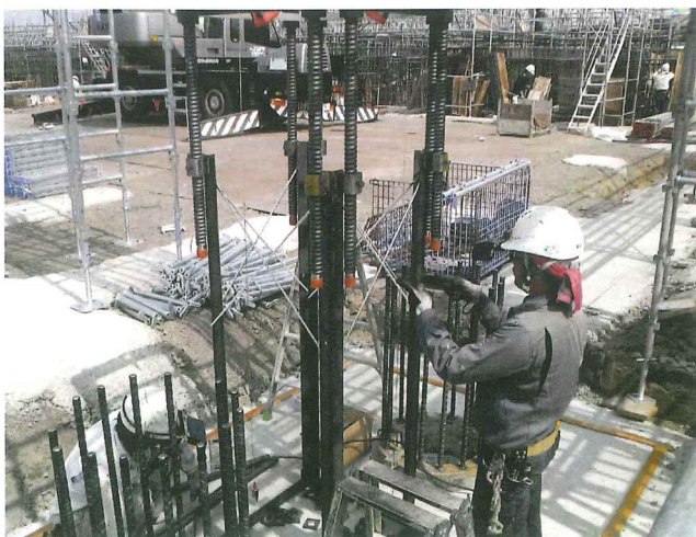
固定柱脚（ベースパック）施工
